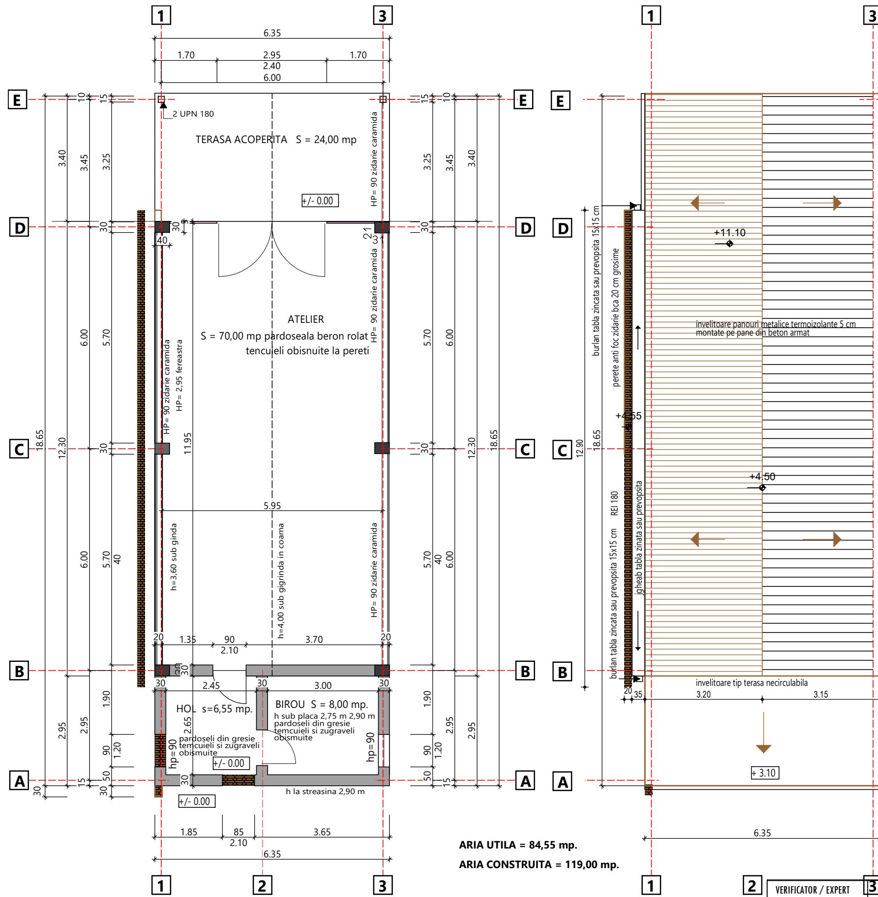
PLAN INVELITOARE
